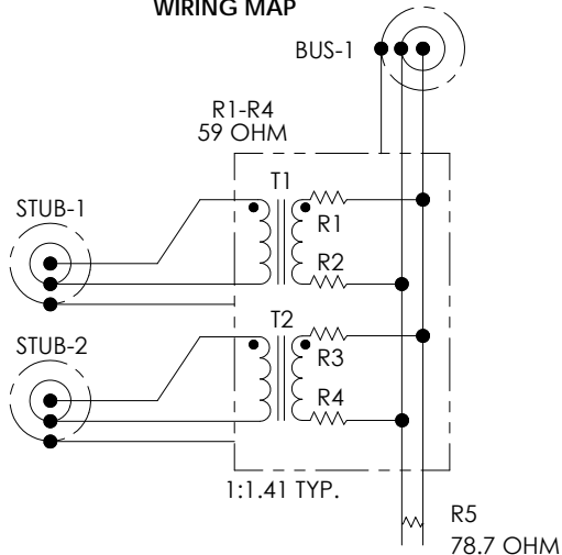
WIRING MAP
