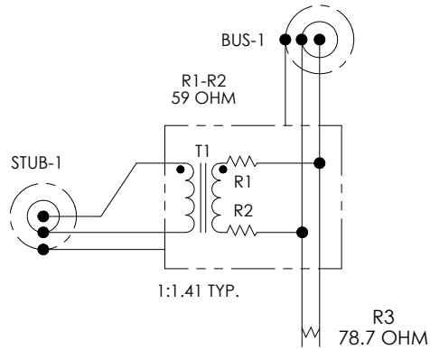
WIRING MAP
