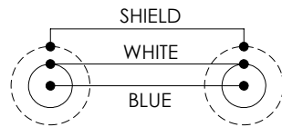
WIRING MAP
