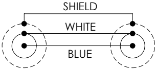
WIRING MAP
