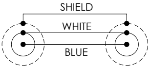
WIRING MAP
