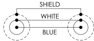
WIRING MAP
