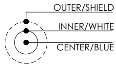
WIRING MAP
