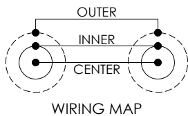
WIRING MAP
