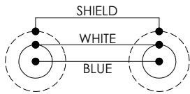
WIRING MAP
