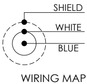
WIRING MAP
