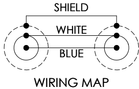
WIRING MAP
