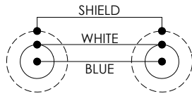
WIRING MAP
